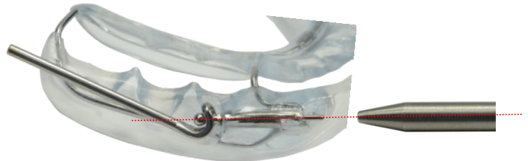
② Mettre la tige-butée dans le système et insérer l'ensemble dans le tube d'armature.
